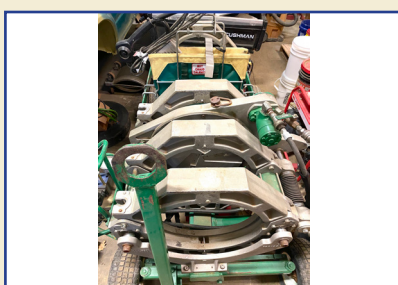
MC ELROY 618 FUSION MACHINE.
